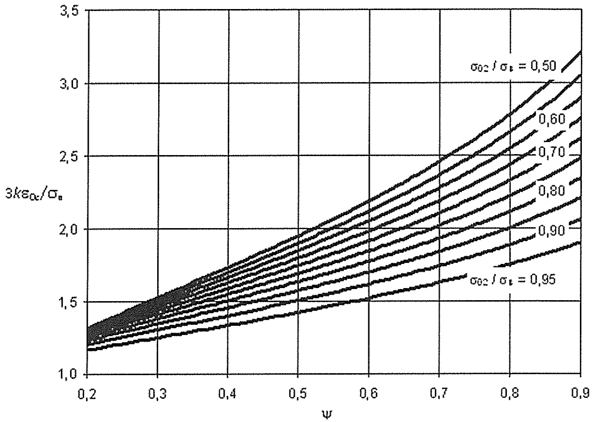
Рисунок 7 – Определение разрушающей объемной деформации \varepsilon_{0c}
